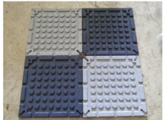
使用X連結器工法-底部示意圖
